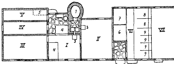
Gammelt 2-Hestes Avl paa Smaalyngen i Aaker. Opmaalt 1928 af H. Zangenberg og K. Thorsen, siden ombygget.
