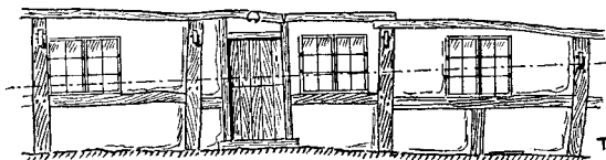
Bindingsværk paa skraat faldende Terræn. »Blæsbyergs« i Østermarie. Opmaalt 1918 af K. Thorsen. Nedbrudt ca. 1920. ----- Vandret Linie.
