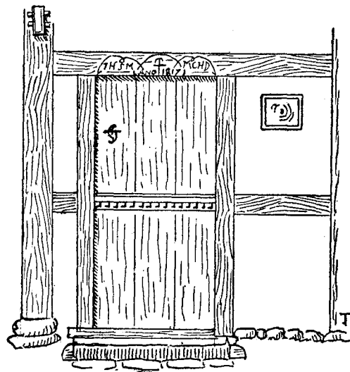
Gl. Indgangsdør paa Husmandsbruget „Toft“ i Knudskeer. Opmaalt 1917 af K. Thorsen
